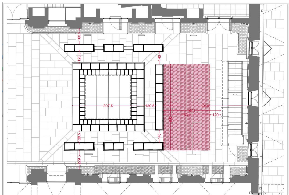
Planimetria n.3
